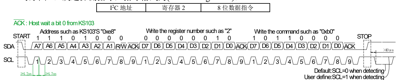
时序图 2: 执行完时序图 1 后, 等待 SCL 变高或延时 100ms 后接收 16 位数据, 先高位后低位, 指令格式为:
