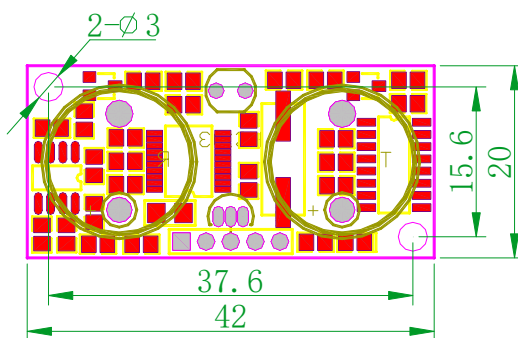
KS103-485 PCB:
