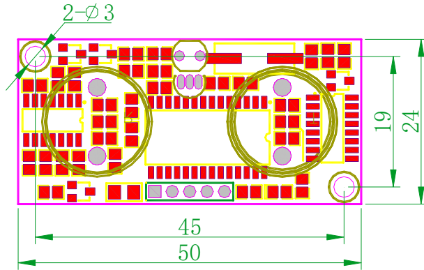
KS103/KS103S PCB:
