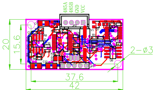
KS103-485 PCB:
